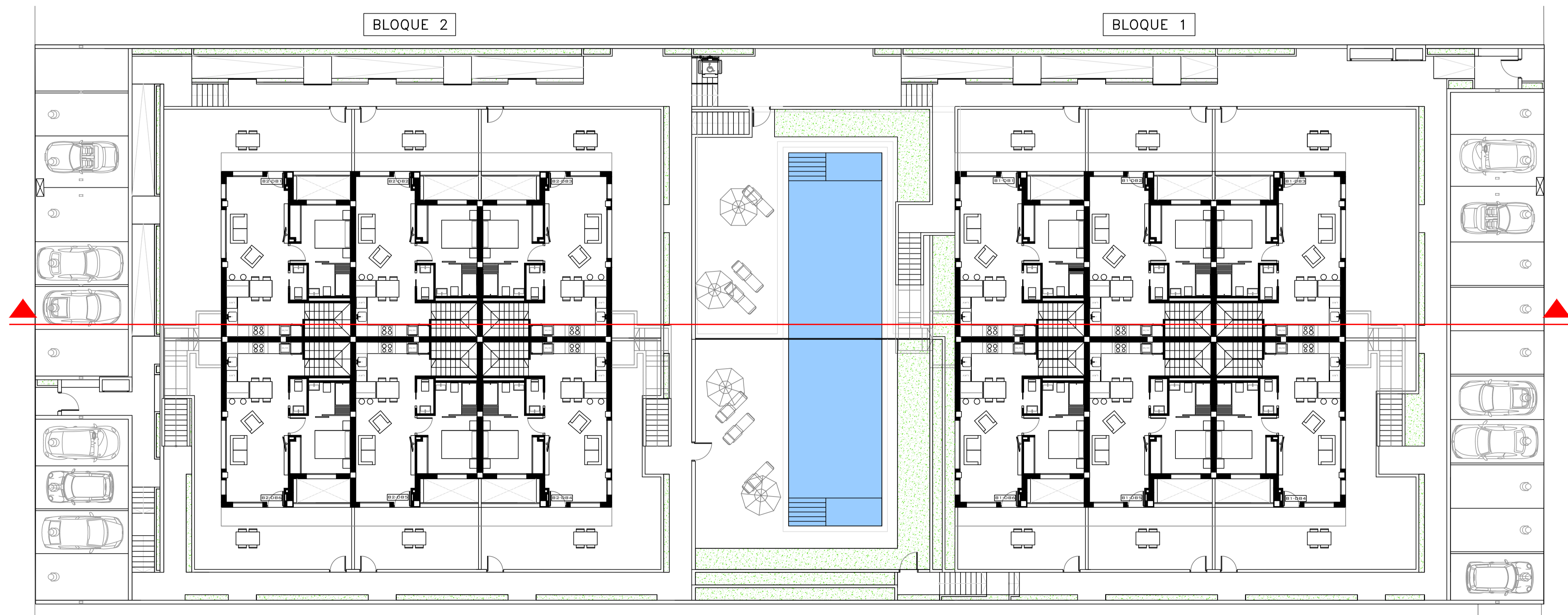
PLANTA BAJA
